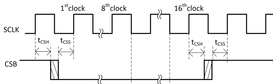
图1 SPI时序图
