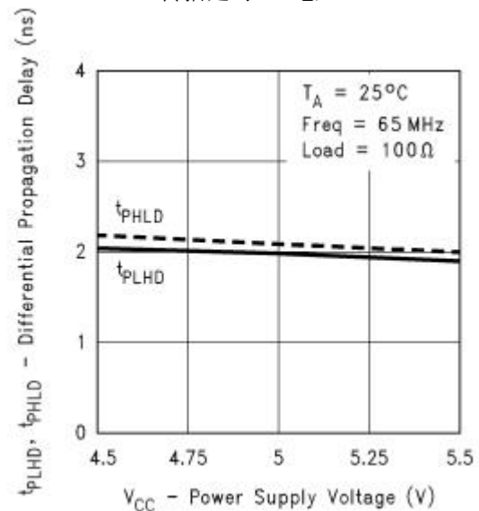
传播延时 VS 电压:
